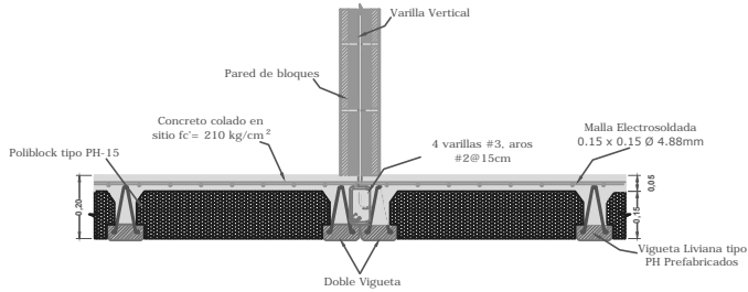
Detalle de Doble vigueta
