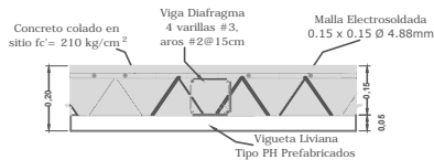
Detalle de Viga Diafragma
