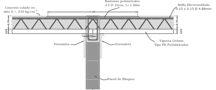
Detalle de Viga Intermedia
