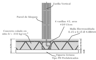
Det. Apoyo de Pared en Viga Diafragma
